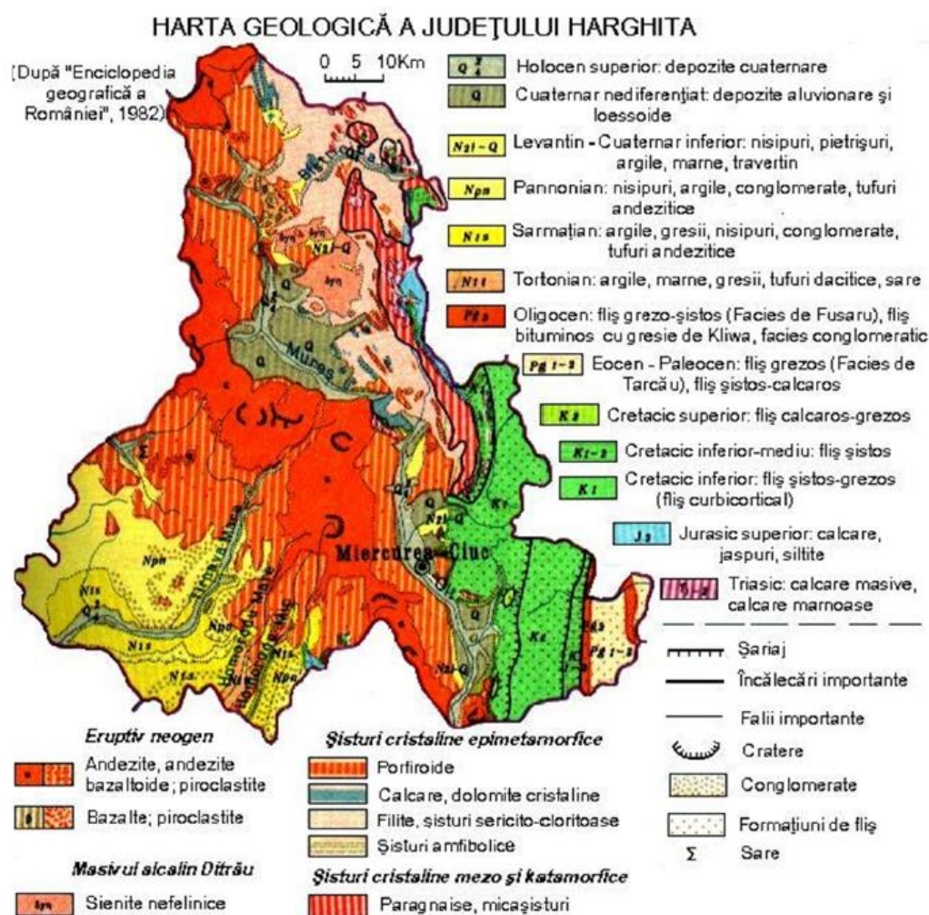
Figura 8 Harta geologică a județului Harghita
