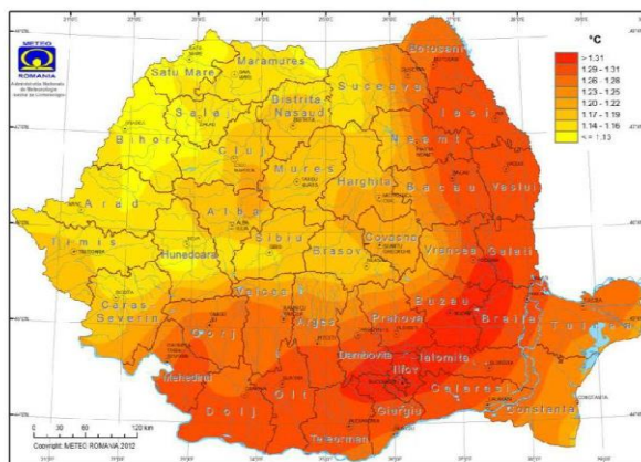
Schimbările medii anuale survenite în temperatura aerului (2011-2040 vs. 1916-1990) (°C)
